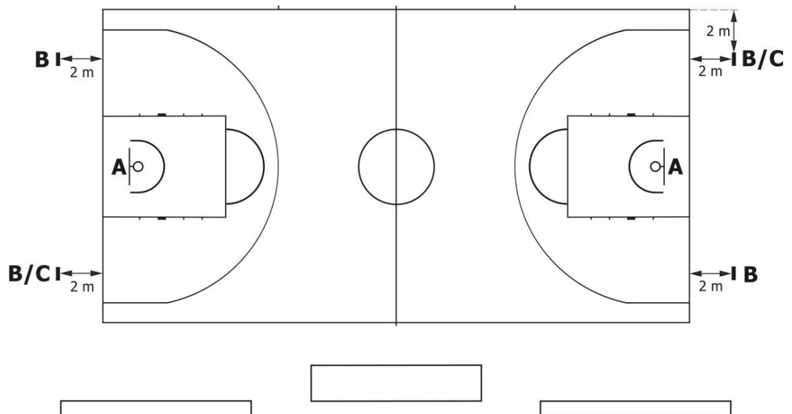
Bild 3.1 Anordnung der Wurfuhr-Anzeigergeräte
